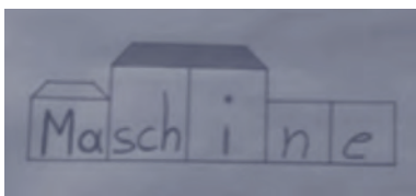
Abb. 9: Auftaktwörter
