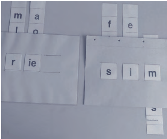
Abb. 8: Silbenschieber blau/rot
